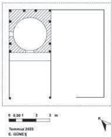
Çizim 9. Mehmet Bircan Fırını planı
