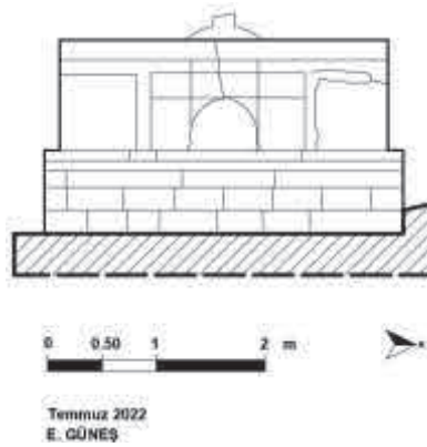
Çizim 24. Muhittin ve Melek Şensoy Fırını ana yapı ön cephe görünüşü
