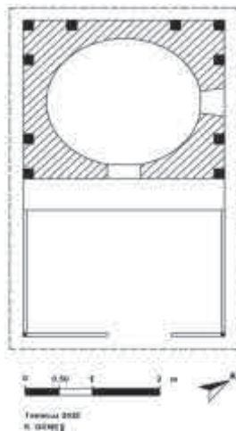
Çizim 20. Sabahattin Somuncu Fırını planı
