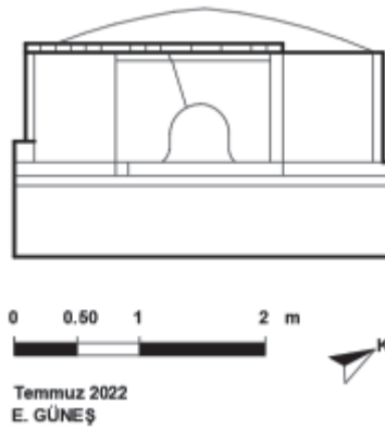
Çizim 6. İsmet Şensoy Fırını ana yapı (pişirme hücresi) ön cephe görünüşü
