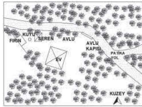
Çizim 16. Cemal Bal Fırını konum plan krokisi
