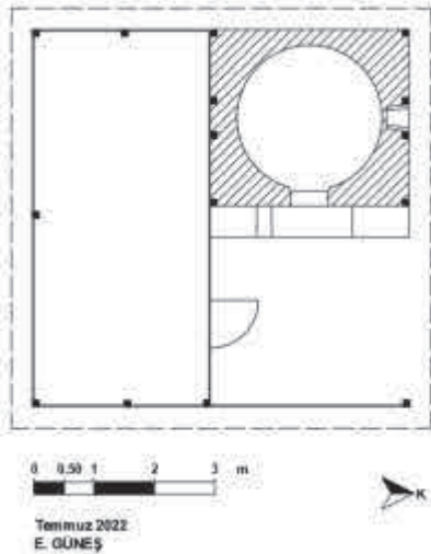
Çizim 23. Muhittin ve Melek Şensoy Fırını planı
