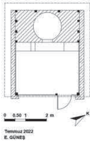
Çizim 5. İsmet Şensoy Fırını planı
