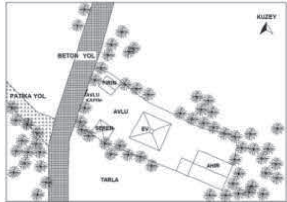
Çizim 4. İsmet Şensoy Fırını konum plan krokisi
