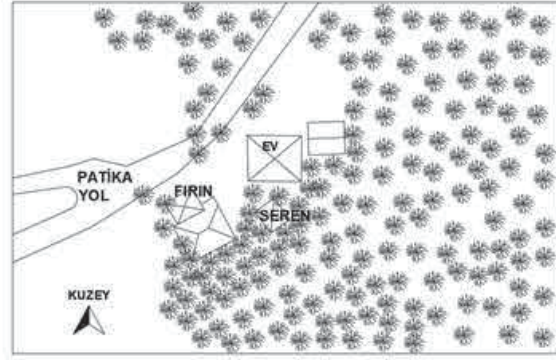
Çizim 26. Resul Zengin Fırını konum plan krokisi
