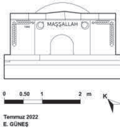
Çizim 10. Mehmet Bircan Fırını ana yapı ön cephe görünüşü
