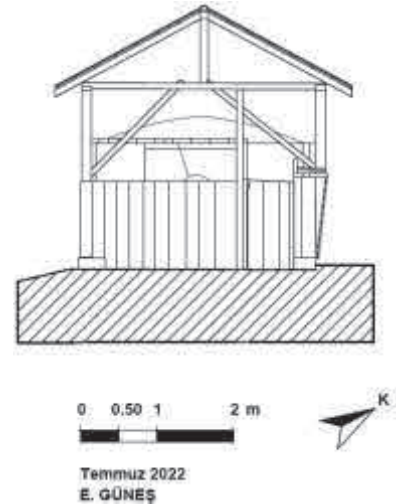
Çizim 7. İsmet Şensoy Fırını ön cephe görünüşü
