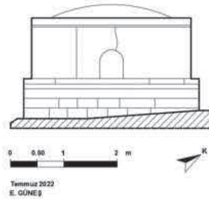
Çizim 21. Sabahattin Somuncu Fırını ana yapı ön cephe görünüşü
