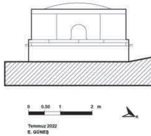
Çizim 28. Resul Zengin Fırını ana yapı ön cephe görünümü
