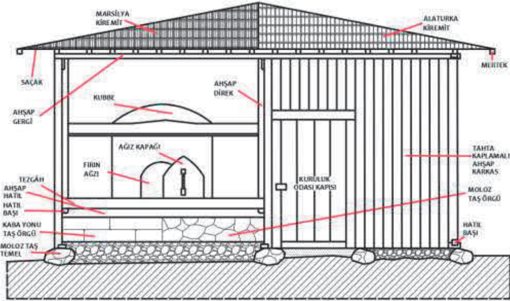
Çizim 3. Şematik ön cephe görünümü üzerinde Alan Köyü fırınlarının bölümleri
