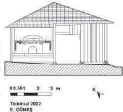
Çizim 11. Mehmet Bircan Fırını ön cephe görünüşü
