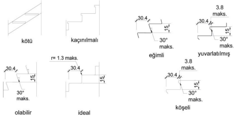
Şekil 1. Merdiven Basamak Ölçüleri (T.C. Aile ve Sosyal Politikalar Bakanlığı, 2011).
