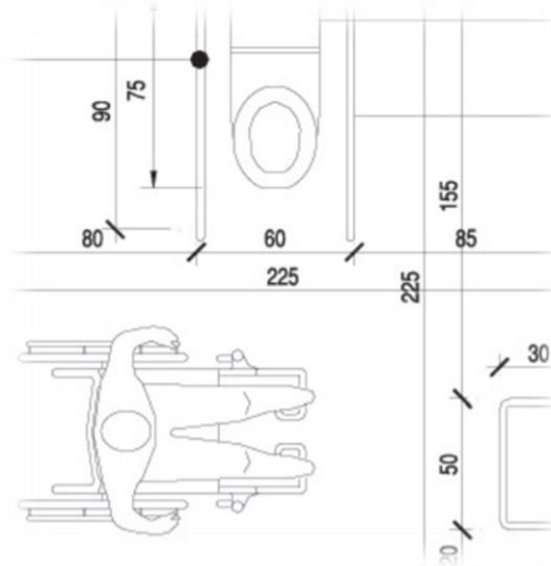
Şekil 2. Engelli Tuvaleti Ölçüleri (T.C. Aile ve Sosyal Politikalar Bakanlığı, 2011).
